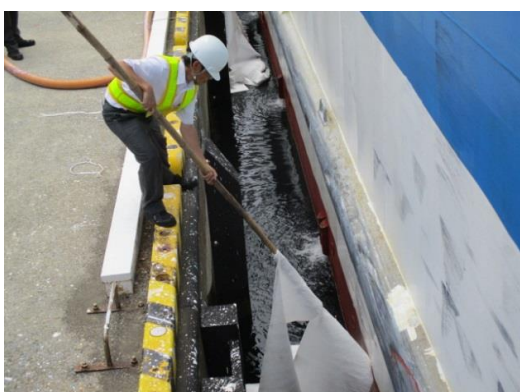
吸着マットで流出油回収
