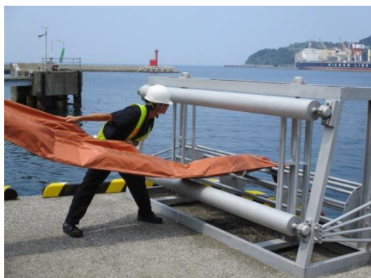
オイルフェンスの送り出し
